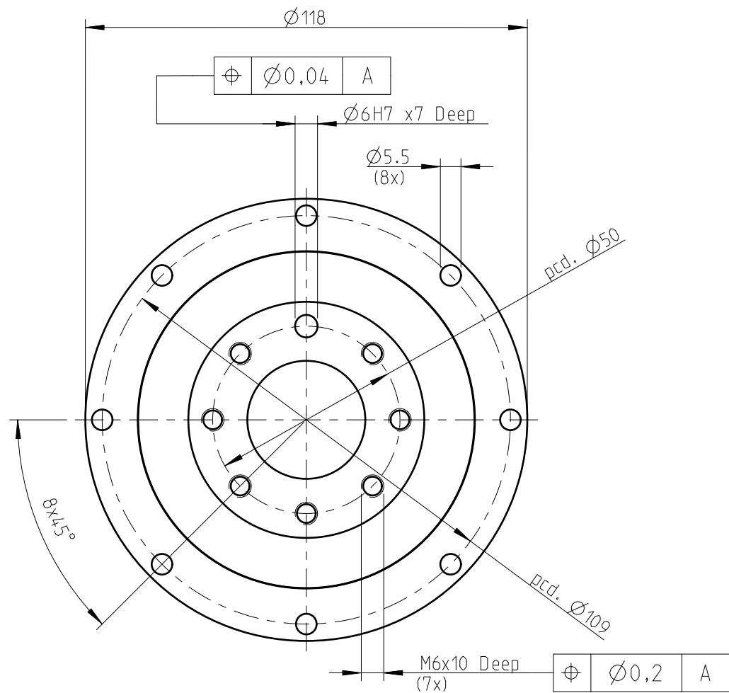
Flange output shaft with dowel hole (EN ISO 9409-1)
