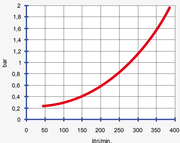
Diagramma perdite di carico Loss of pressure diagram
