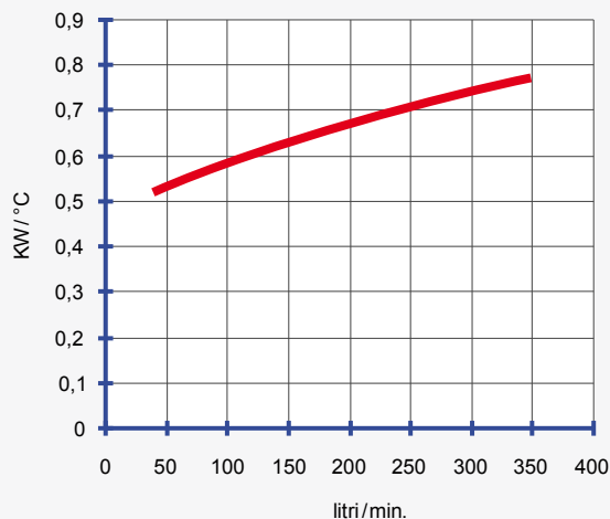
Diagramma di rendimento Performance diagram
