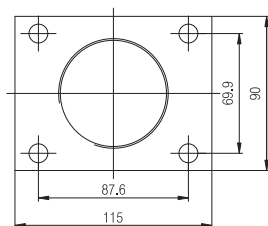
Rectangular Flange(LA64-RF)
