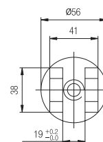
Rod Clevis(LA64-RC)
