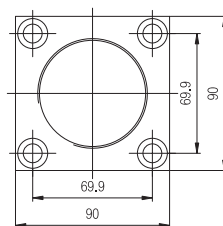
Square Flange(LA64-SF)
